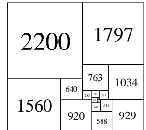
17 : 3997x3760A
