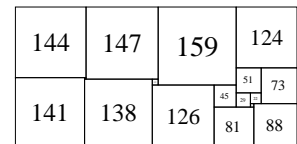
17 : 574x285A
