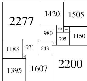
17 : 5202x4855A
