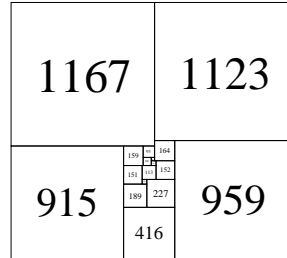
17 : 2290x2082A
