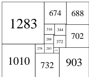
17 : 2645x2293A
