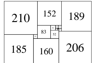
17 : 551x395A
